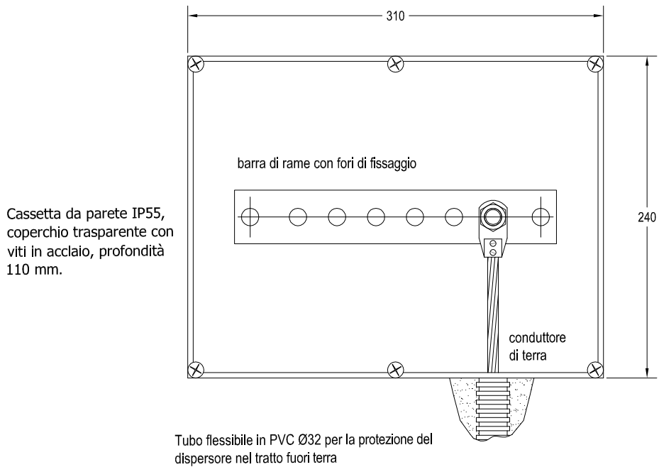
VISTA FRONTALE
