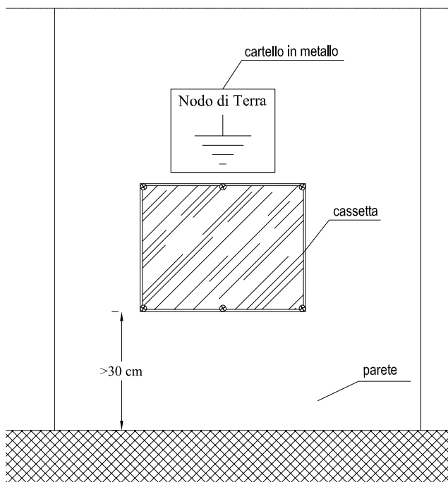
POSIZIONE CASSETTA
