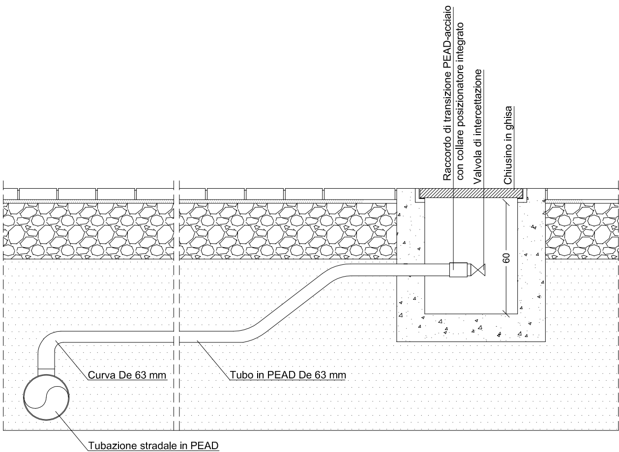
SEZIONE
